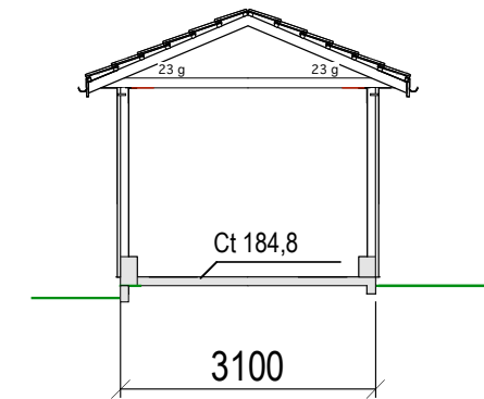
SNITT
